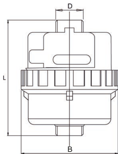
Dimensiones RNK-L-RP-N
